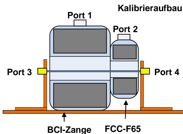
Abbildung 6: Kalibrierenaufbau für De-embedding der Messstruktur (links). Gemessene Transmission zwischen den vier Ports im Kalibrierenaufbau (rechts)
