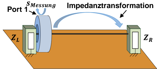
Abbildung 3: Reflexionsmessung mit BCI-Zange
