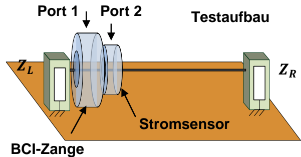
Abbildung 5: Positionierung der Sensoren in einem Testaufbau
