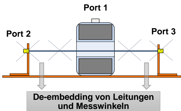
Kalibrieraufbau
